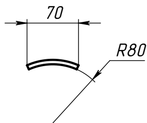
Поз.7 (Накладка)
